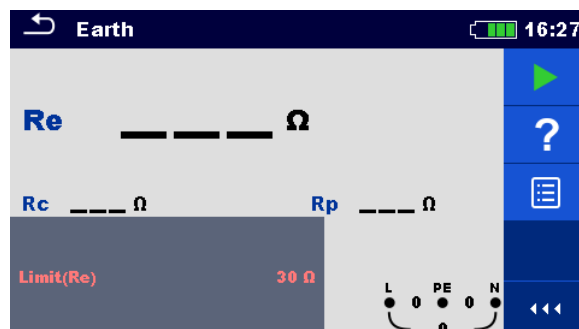
Abbildung 4.46 Menü Erde 3-Leiter
