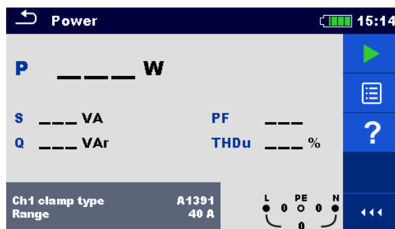
Abbildung 4.53: Menü Leistung
