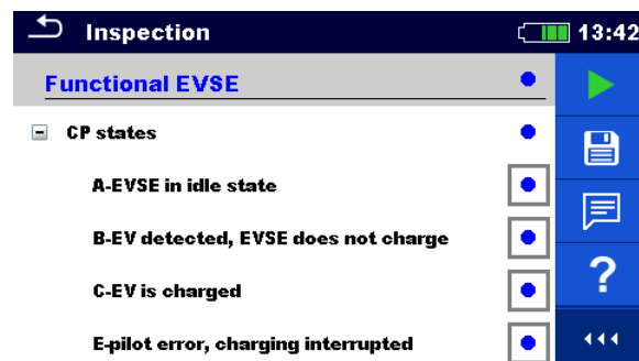
Abbildung 4.86: Beispiel für ein Ergebnis der Funktionsprüfung
