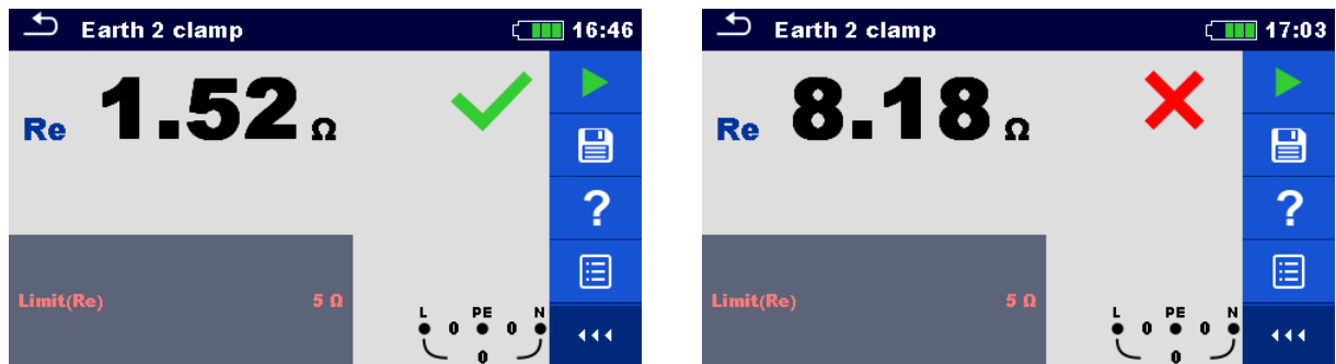
Abbildung 4.52: Beispiele für Ergebnisse der Erdungsmessung mit 2 Stromzangen
