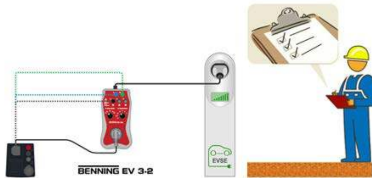
Abbildung 4.85: Funktionsprüfung
