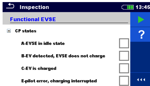
Abbildung 4.84: Beispiel für das Menü Funktionsprüfung
