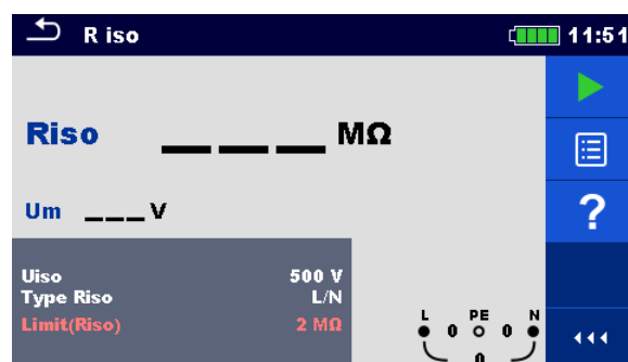
Abbildung 4.6: Menü Isolationswiderstandsmessung
