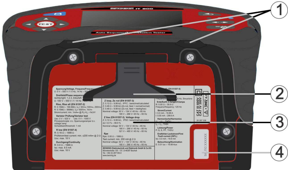
Abbildung 2.5: Unterseite
