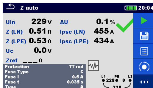
Abbildung 4.45: Beispiele für Ergebnisse der Z Auto Messung
