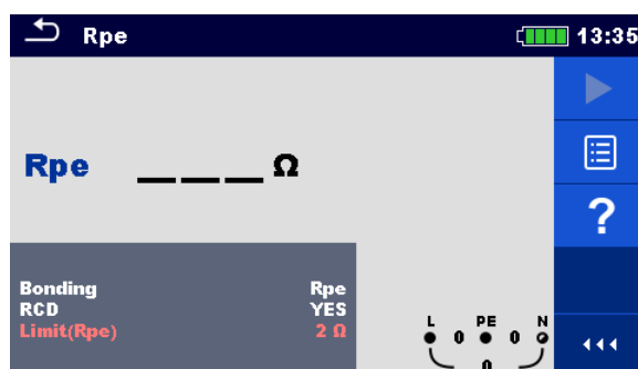
Abbildung 4.66: Menü Schutzleiterwiderstand
