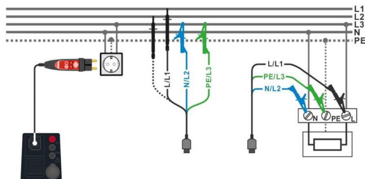
Abbildung 4.79: AUTO TN-Messung
