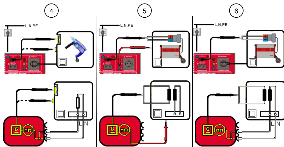
Abb. 8: Isolationswiderstand prüfen SK II (Anschlussschema beispielhaft für VDE 0701 und VDE 0702, Stromlaufplan)
