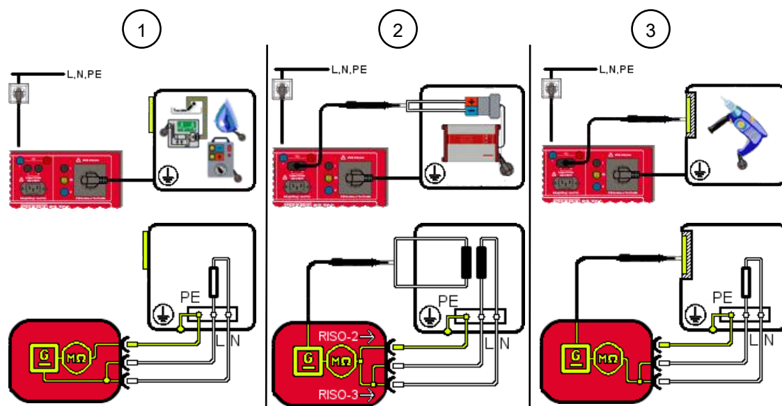
Abb. 7: Isolationswiderstand prüfen SK I (Anschlussschema beispielhaft für VDE 0701 und VDE 0702, Stromlaufplan)
