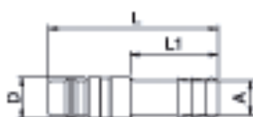
Einstecktülle
