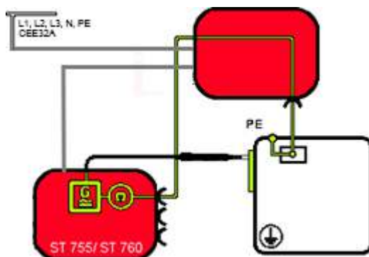
Stromlaufplan
