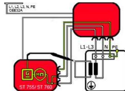
Stromlaufplan
