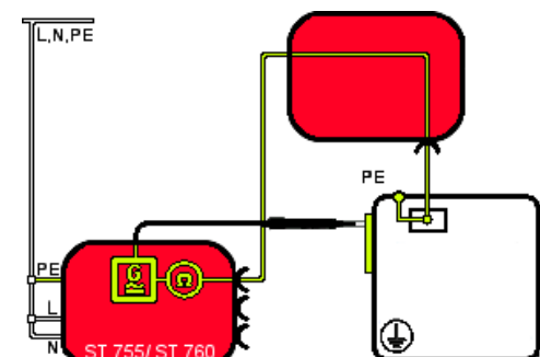
Stromlaufplan
