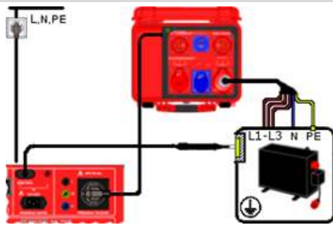
Anschlusschema
