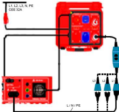
Anschlusschema PRCD
