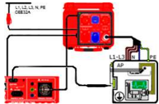
Anschlusschema
