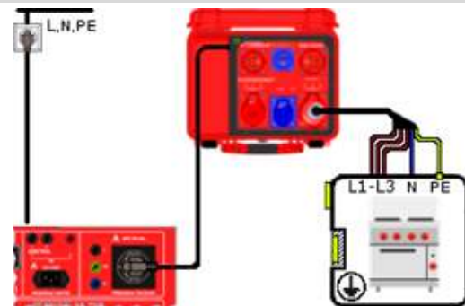
Anschlusschema
