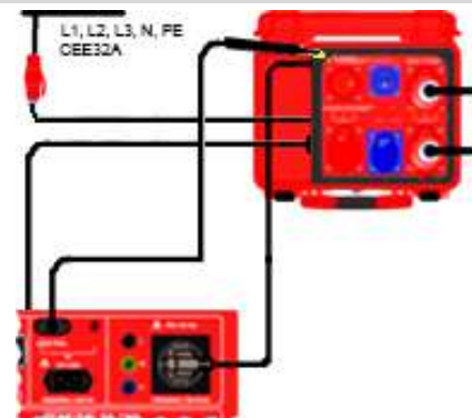
Anschlussschema
