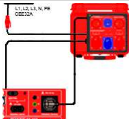
Anschlusschema
