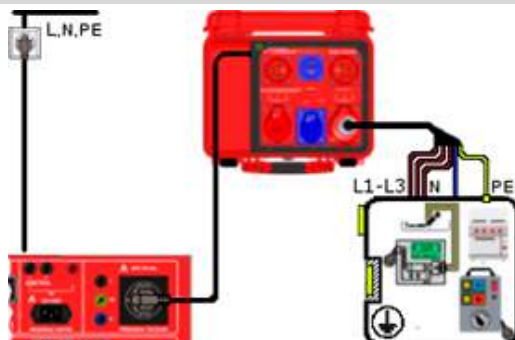
Anschlusschema
