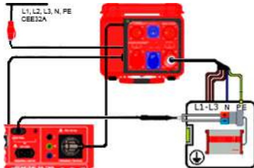
Anschlussschema
