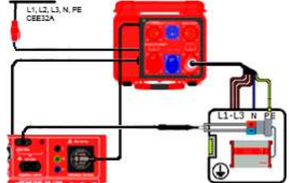
Anschlussschema
