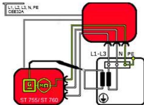
Stromlaufplan
