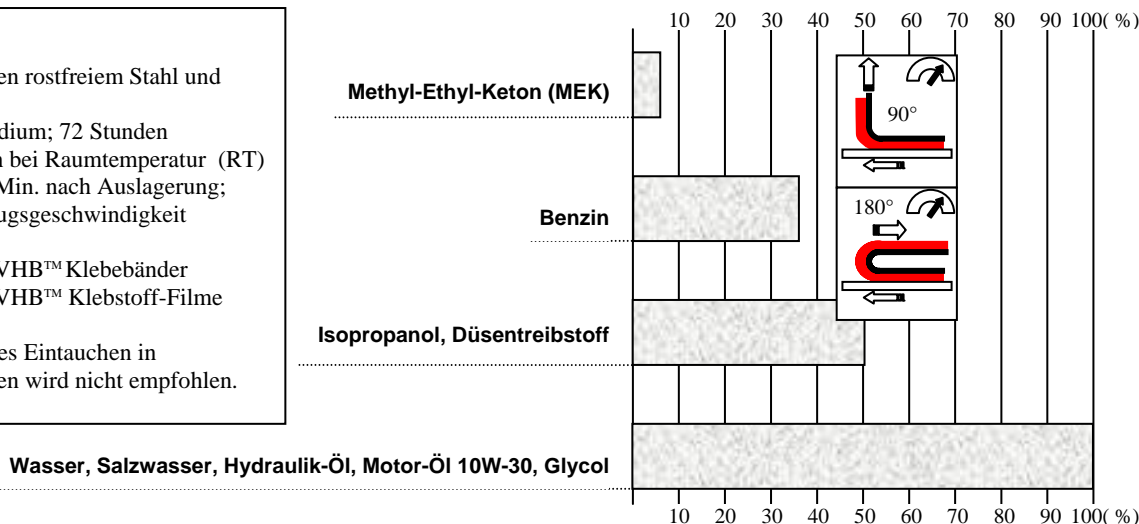
Diagramm 2: Lösemittelbeständigkeiten VHB™ Klebebänder
