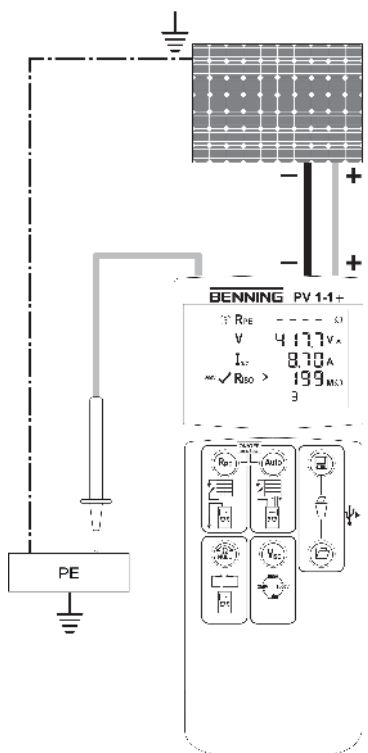
Abb. 5: Automatische PV-Messung
