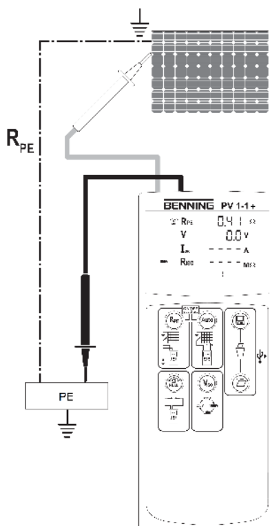
Abb. 4: Schutzleiterwiderstand
