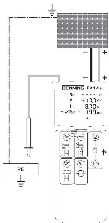
Abb. 8: Automatische PV-Messung
